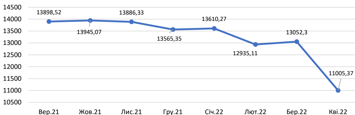
Графік 8. Фонд національного добробуту рф млрд руб.
